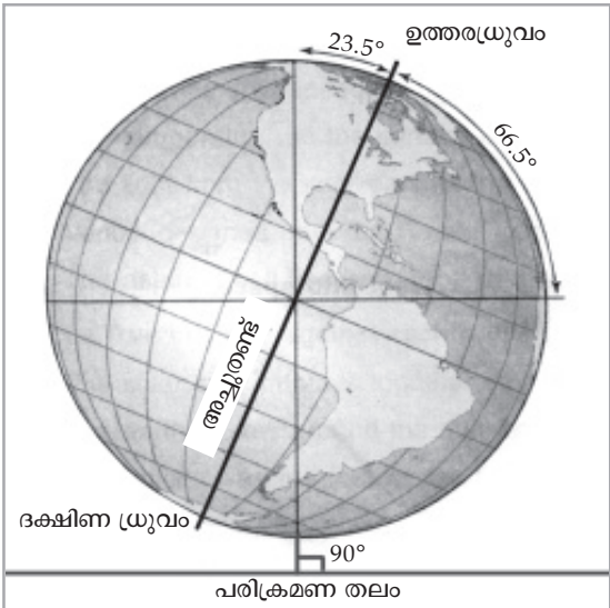
ഭൂമിയുടെ ചരിവ് ഡിഗ്രിയിൽ
